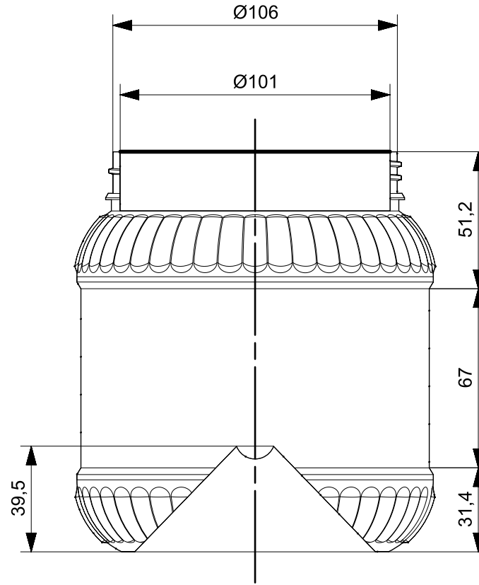
SECTION A-A
